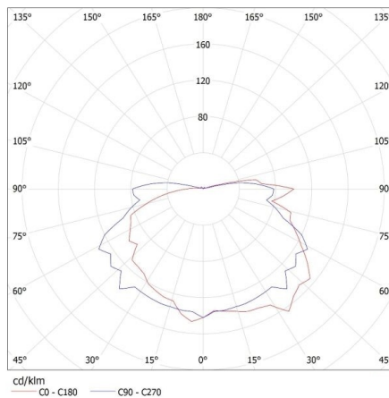
KANLUX S.A. (kat 4260) TUNA S1101 / Krzywa rozsyłu światła (biegunowo)
