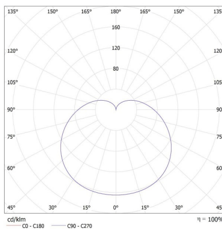
KANLUX S.A. (kat 33724) IQ-LEDDIM A60 10,5W-WW / LDC (Polar)
