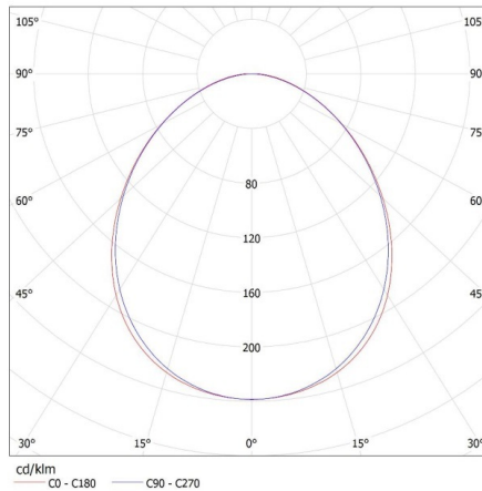
KANLUX S.A. (kat 27414) ALIN 4LED 1X120-B + GLASSv4 / LDC (Polar)
