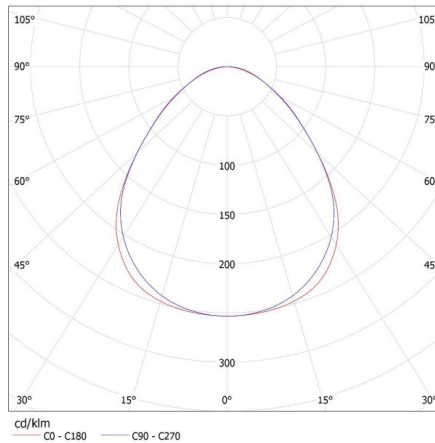
KANLUX S.A. (kat 28455) AL 4LED 150-MPR-W + GLASSv4 / LDC (Polar)
