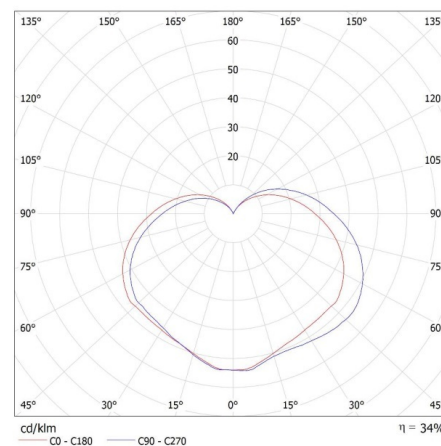
KANLUX S.A. (kat 36546) LAVEN 50 GR + IQ-LED / LDC (Polar)
