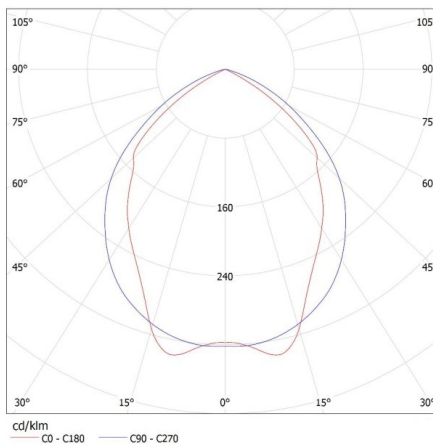
KANLUX S.A. (kat 22673) REGIS 4LED 418 PT + T8 Miledo / Krzywa rozsyłu światła (biegunowo)
