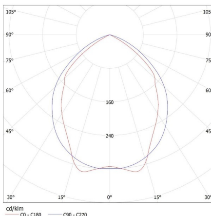
KANLUX S.A. (kat 22673) REGIS 4LED 418 PT + T8 Miledo / Krzywa rozsyłu światła (biegunowo)
