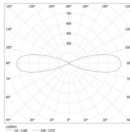
KANLUX S.A. (kat 22441) ZEW EL-235U-B + IQ-LED ... 7W S3 / LDC (Polar)
