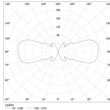
KANLUX S.A. (kat 22441) ZEW EL-235U-B + IQ-LED ... 7W / LDC (Polar)
