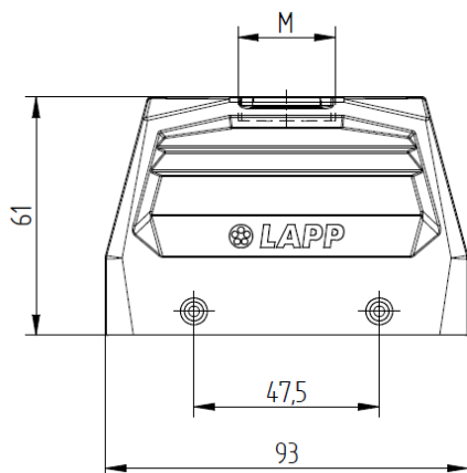
Kabeleingang gerade
