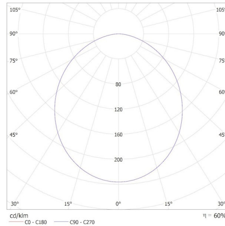
KANLUX S.A. (kat 39022) DABER 8-13W CCT B 13W / Krzywa rozsyłu światła (biegunowo)
