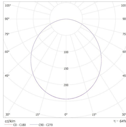
KANLUX S.A. (kat 39024) DABER 12-20W CCT W 20W / Krzywa rozsyłu światła (biegunowo)
