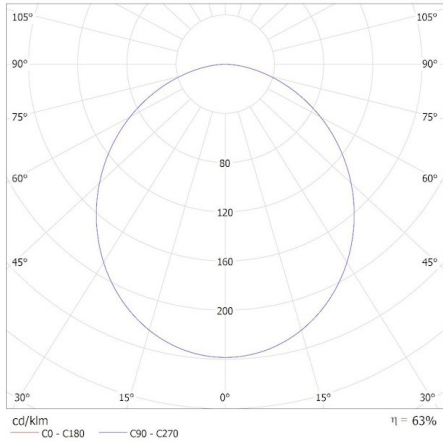
KANLUX S.A. (kat 39026) DABER 12-20W CCT B 20W / Krzywa rozsyłu światła (biegunowo)
