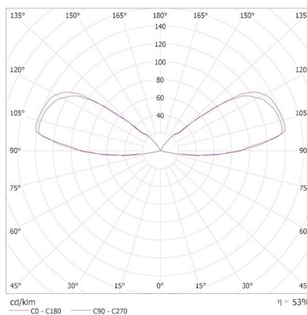
KANLUX S.A. (kat 39180) REFAZI EL 6W-F-W / Krzywa rozsyłu światła (biegunowo)
