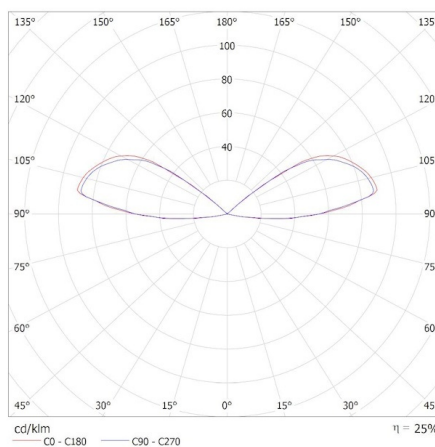
KANLUX S.A. (kat 39181) REFAZI EL 6W-F-GR / Krzywa rozsyłu światła (biegunowo)
