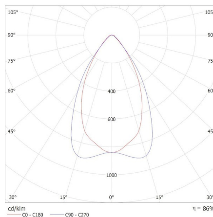
KANLUX S.A. (kat 37545) KNU-S6D-NW-B-P1D / Krzywa rozsyłu światła (biegunowo)
