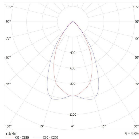
KANLUX S.A. (kat 37538) KNU-M6D-WW-W-P1D / Krzywa rozsyłu światła (biegunowo)
