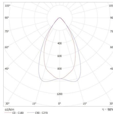
KANLUX S.A. (kat 37539) KNU-S6D-NW-W-P1D / Krzywa rozsyłu światła (biegunowo)
