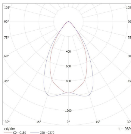
KANLUX S.A. (kat 37540) KNU-L6D-NW-W-P1D / Krzywa rozsyłu światła (biegunowo)
