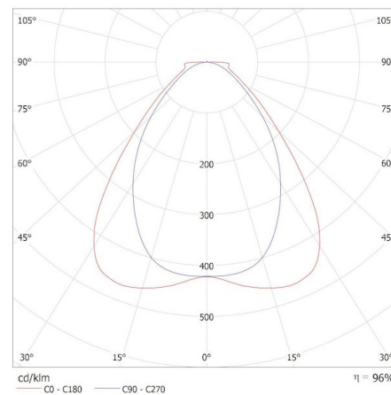
KANLUX S.A. (kat 37449) KN-S9D-NW-W-P1 / Krzywa rozsyłu światła (biegunowo)
