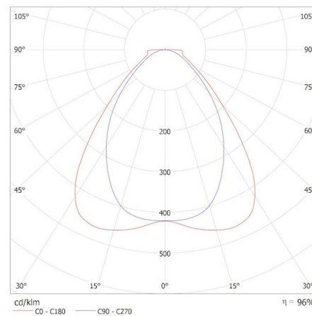
KANLUX S.A. (kat 37451) KN-M9D-NW-W-P1 / Krzywa rozsyłu światła (biegunowo)
