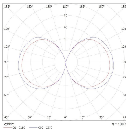
KANLUX S.A. (kat 37386) XLED G45 E14 7W-WW / Krzywa rozsyłu światła (biegunowo)
