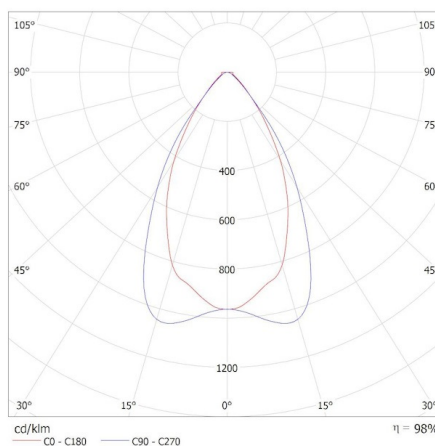
KANLUX S.A. (kat 37488) KN-S6D-WW-W-P3 / Krzywa rozsyłu światła (biegunowo)
