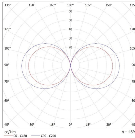
KANLUX S.A. (kat 36542) PRESO 30 GR + XLED / LDC (Polar)
