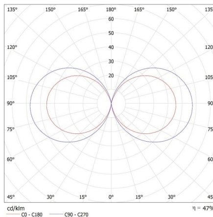
KANLUX S.A. (kat 36542) PRESO 30 GR + IQ-LED / LDC (Polar)
