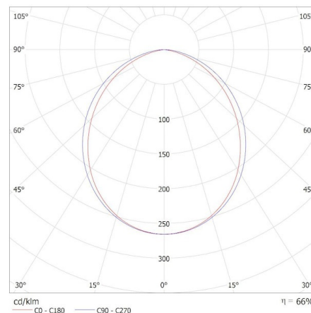
KANLUX S.A. (kat 36371) KXL 24W 2880 90 NW B / Krzywa rozsyłu światła (biegunowo)
