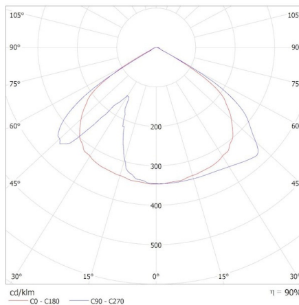
KANLUX S.A. (kat 36435) PARCOLI 30-50W CCT G_45st / Krzywa rozsyłu światła (biegunowo)
