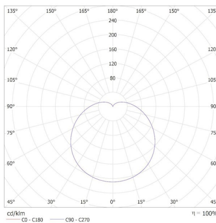
KANLUX S.A. (kat 36697) IQ-LED G45E27 5,9W-WW / Krzywa rozsyłu światła (biegunowo)
