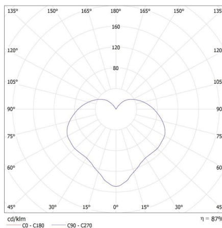
KANLUX S.A. (kat 36534) LIEGO 37 B + IQ-LED / LDC (Polar)
