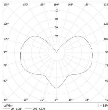
KANLUX S.A. (kat 36534) LIEGO 37 B + XLED / LDC (Polar)
