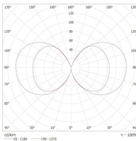
KANLUX S.A. (kat 33099) XLED A60 4,5W-NW / Krzywa rozsyłu światła (biegunowo)
