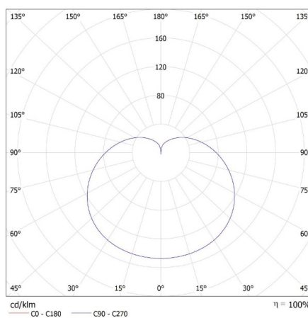
KANLUX S.A. (kat 33746) IQ-LED A67 N 19W-WW / LDC (Polar)
