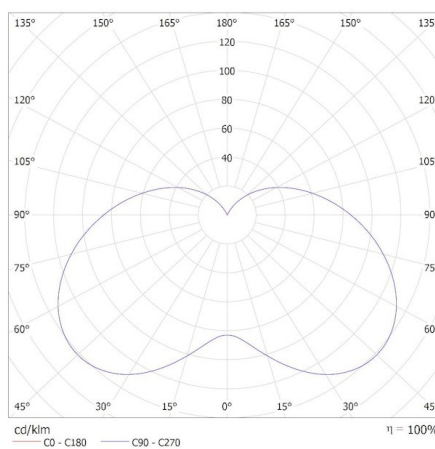
KANLUX S.A. (kat 23437) DUN 6,5W E14-WW / Krzywa rozsyłu światła (biegunowo)
