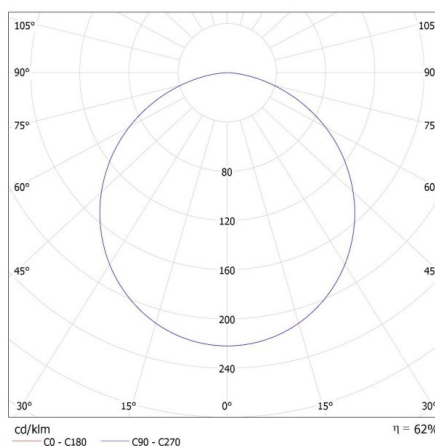
KANLUX S.A. (kat 35662) BTLW 18W-930-W / LDC (Polar)
