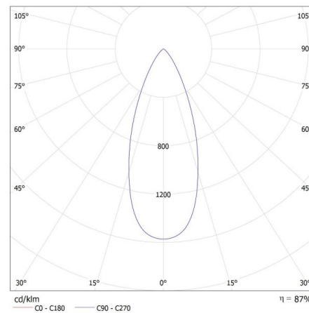
KANLUX S.A. (kat 36561) USTI SP 1X7 GR + IQ-LED ... 6,5W-S3 / LDC (Polar)
