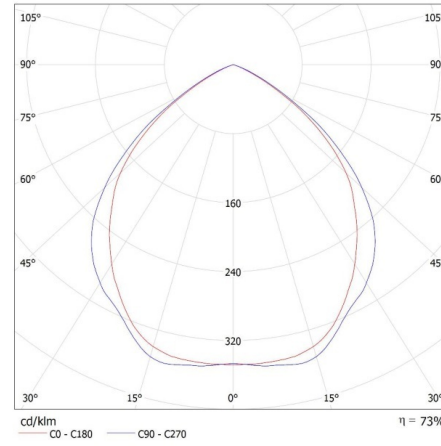
KANLUX S.A. (kat 36561) USTI SP 1X7 GR + IQ-LED ... 6,5W / LDC (Polar)
