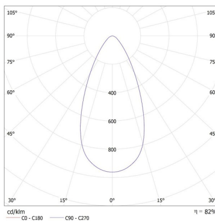
KANLUX S.A. (kat 35654) BTL 28W-930-W 45deg / LDC (Polar)
