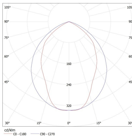
KANLUX S.A. (kat 25711) NOTUS 3WS EVG 418 NT / Krzywa rozsyłu światła (biegunowo)
