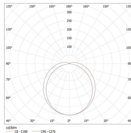
KANLUX S.A. (kat 28866) FTHL1500 73W-840-OPL / LDC (Polar)
