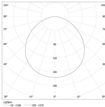
KANLUX S.A. (kat 23124) JASMIN 370-W + IQ-LED / LDC (Polar)
