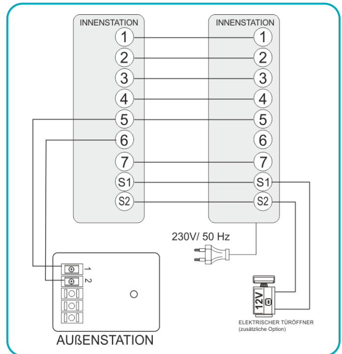
Abb. 4 Schaltplan OR-DOM-RL-902
