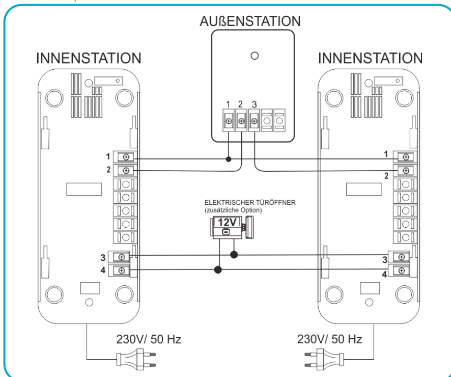
Abb. 5 Schaltplan OR-DOM-RL-903
