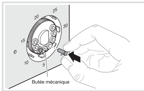
Ex : blocage de la consigne à 20 °C
